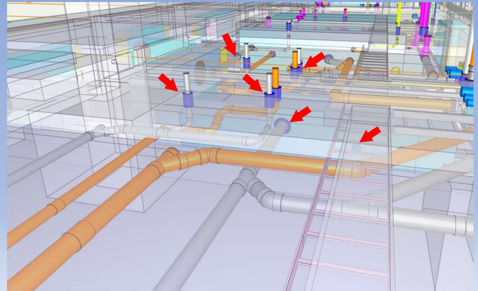
地中梁スリーブ スラブ・壁スリーブなど
